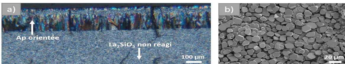
Figure 1. a) Micrographie optique en lumière polarisée du produit de réaction formé par la diffusion entre \text{La}_2\text{SiO}_5 / \text{SiO}_2 après frittage réactif à 1600^\circ\text{C}/10\text{h} . b) Cristaux d'oxyapatite orientés. © IRCER
