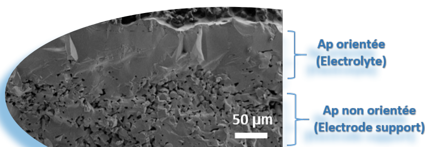
Figure 2. Micrographie MEB de la section transversale de la fracture du bicouche \text{La}_2\text{SiO}_5 / \text{SiO}_2 après frittage réactif à 1600^\circ\text{C}/10\text{h} . © IRCER
